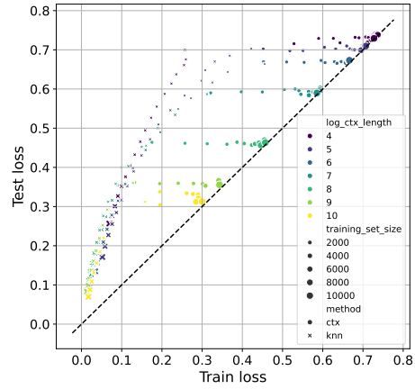
(d) eeg-eye-state
