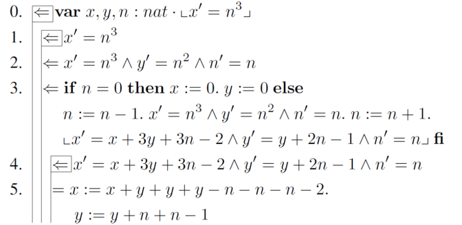
Fig. 6. Refinement
