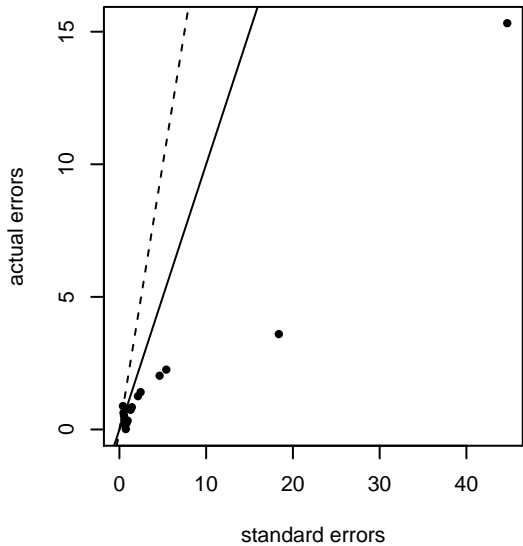
Method nlm Parameter w
