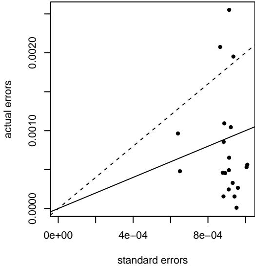
Method nlm Parameter b
