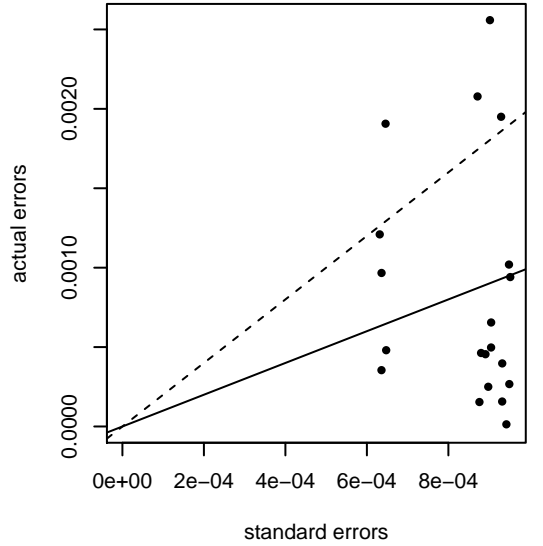
Method optim Parameter b
