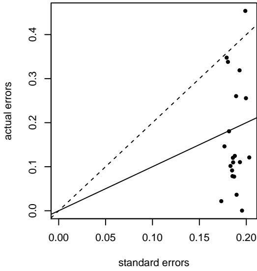
Method nlm Parameter a
