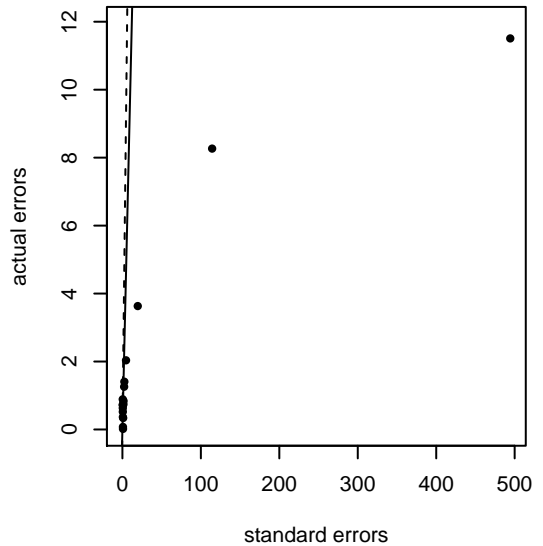
Method optim Parameter w
