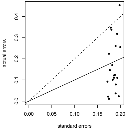
Method optim Parameter a
