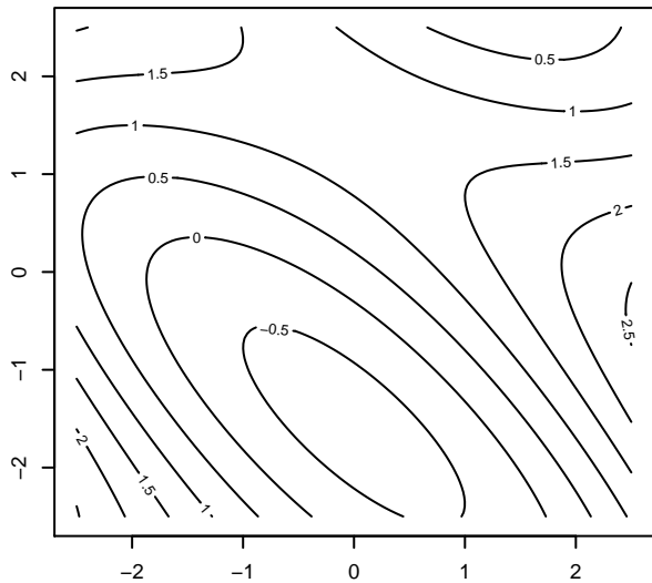
True function
